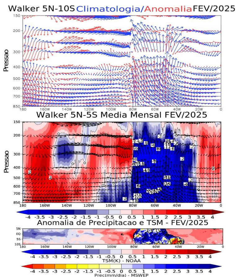
Figura 8. Superior: Climatologia (azul) e anomalia (vermelho) do movimento vertical zonal (entre 5°N e 10°S) em fevereiro de 2025. Centro: Média do movimento vertical observado. Inferior: anomalias de TSM (°K) e precipitação (mm). Dados do CPC/NCEP e MSWEP processados pelo LABCLIM-UEA.
