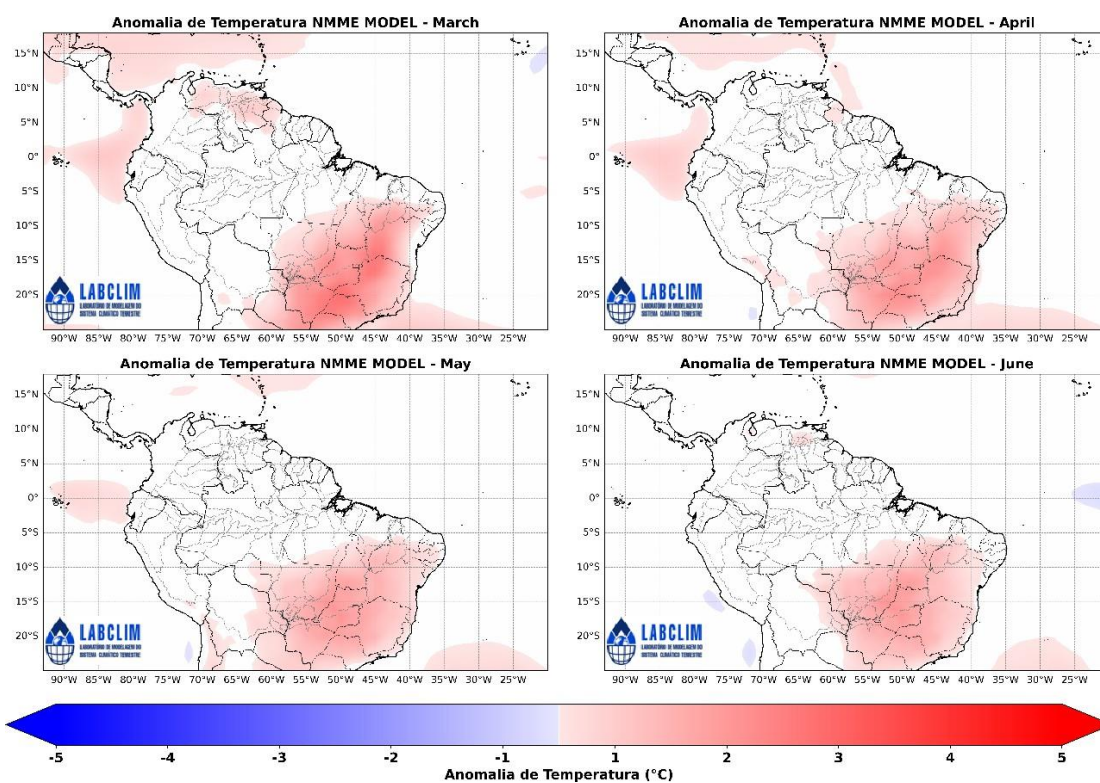
Figura 12. Previsões sazonais de anomalias de Temperatura (°C) do North American Multi-Model Ensemble (NMME) para os meses de março a junho de 2025 (FMAM). Fonte dos dados: NMME.
