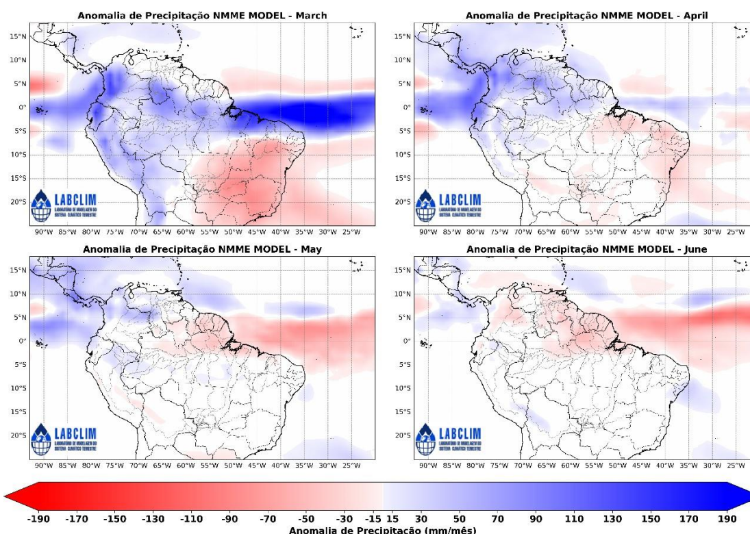
Figura 10. Previsões sazonais de anomalias de precipitação (mm/mês) do North American Multi-Model Ensemble (NMME) para os meses de março a junho de 2025 (MAMJ). Fonte dos dados: NMME.
