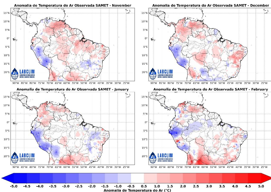
Figura 9. Anomalia de Temperatura do Ar a 2m (°C) na bacia Amazônica para os meses de novembro de 2024 a fevereiro de 2025, provenientes do produto South American Mapping of Temperature (SAMET).
